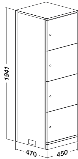
Kovová varianta
